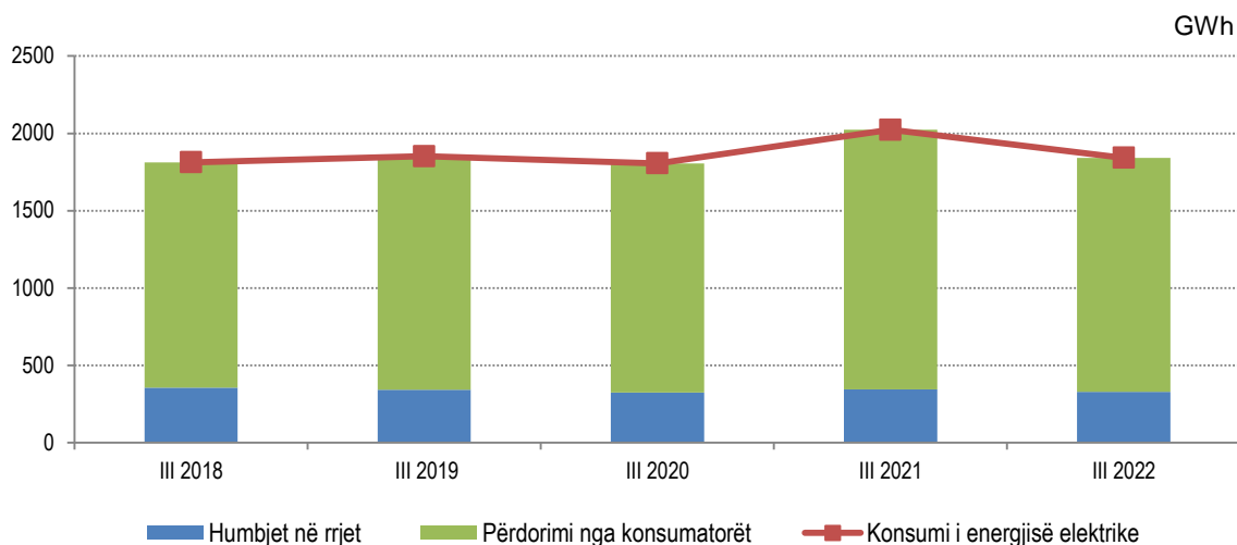
Fig. 3 Konsumi i energjisë elektrike, humbjet në rjet dhe përdorimi nga konsumatorët
