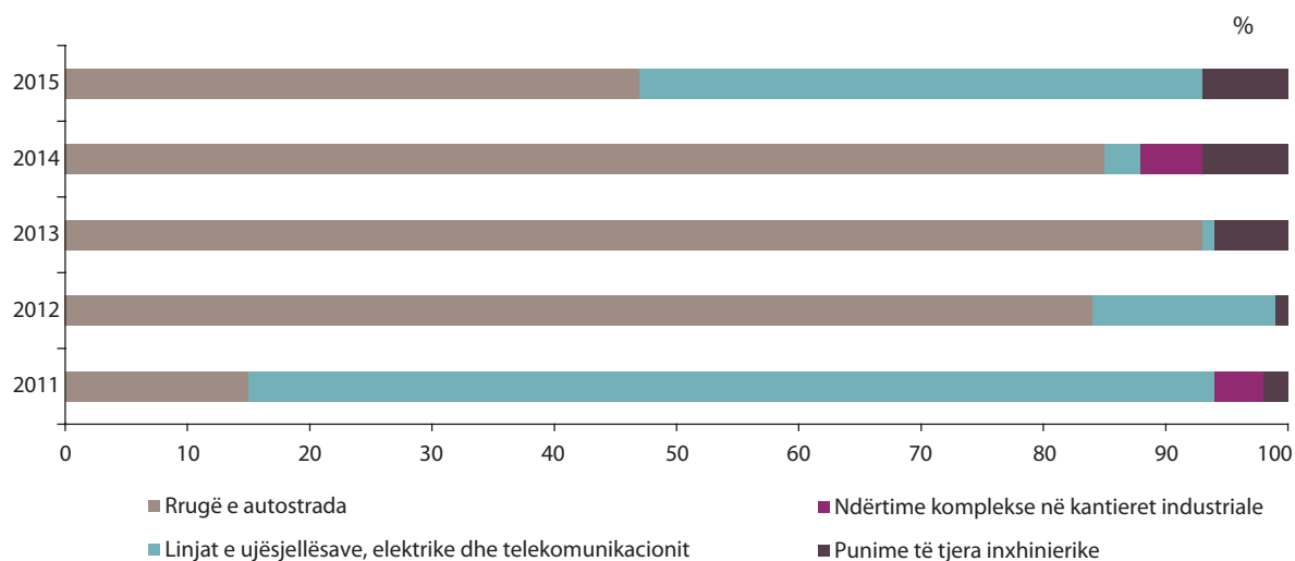
Fig. 5 Struktura e punimeve inxhinierike sipas lejeve të ndërtimit të miratuara
